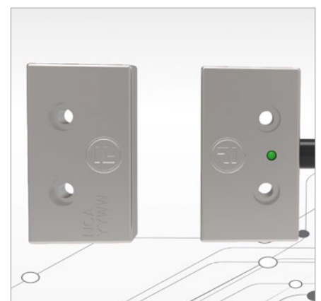
Robustes Design im Edelstahlgehäuse mit LED-Diagnose
